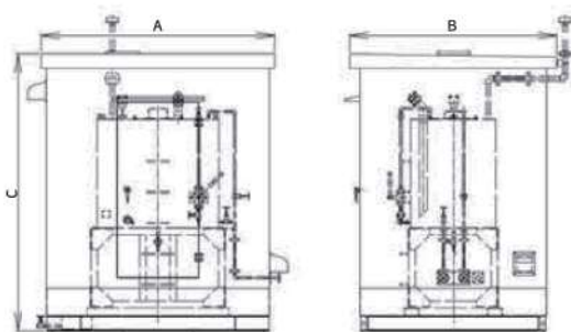
燃料庫
