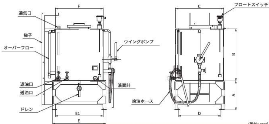
燃料タンク
